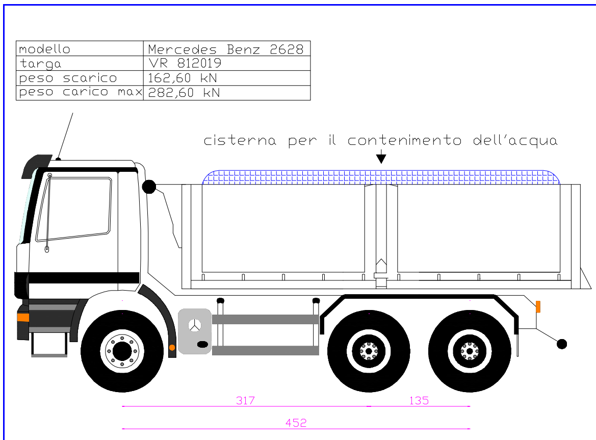
Fig. 3: Caratteristiche dell'automezzo
